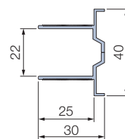
■固定カムチ
