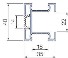
■カムチ
