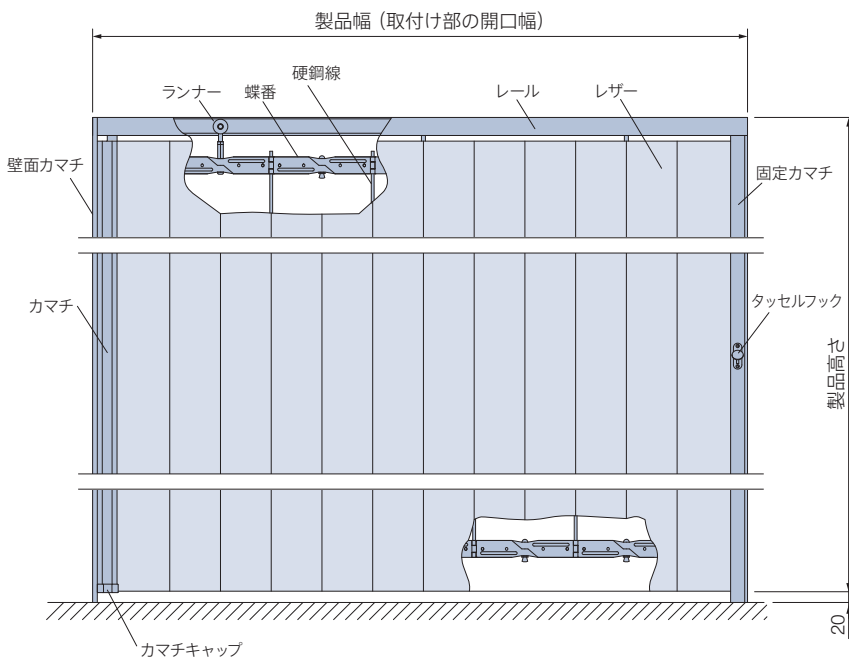
■正面図
