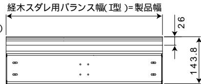
天井付け用 型 (大型タイプの場合の伏せ図)
