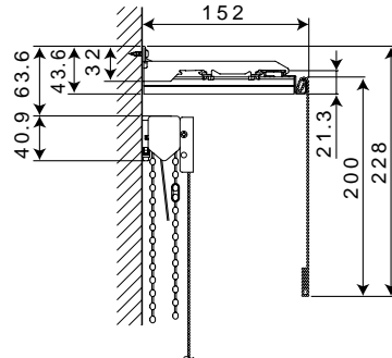
正面付け用 C 型 (大型タイプの場合の伏せ図)
