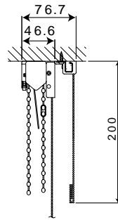
天井付け用 型 (大型タイプの場合の伏せ図)
