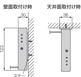
ステー (取付けプレート)
