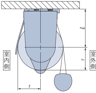
r: 生地の巻取り半径 Q: サイドブラケット FF=49、SS=56
