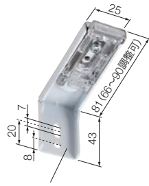
正面付け補助金具(14)
