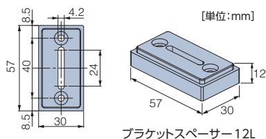
ブラケットスペーサー 12L
