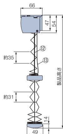
天井付け・正面付け共通
