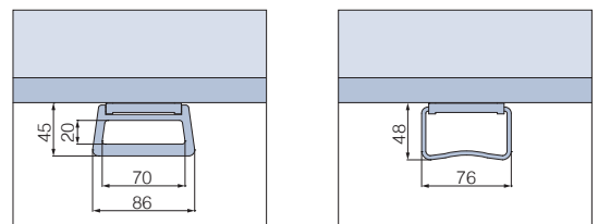
プルハンドル・クリアプルハンドル
