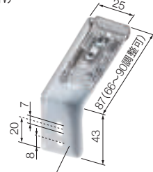
正面付け補助金具 (14)
