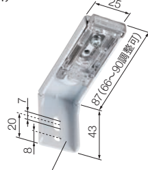
正面付け補助金具 (I4)
