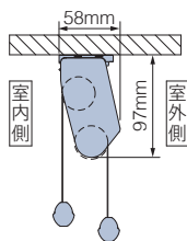
ラルク ダブル小型
