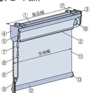
生地が竹スダレの場合 (チェーン操作)
