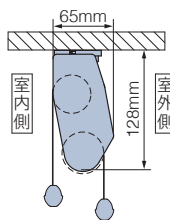
ラルク ダブル
