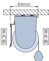
ラルクシールド
