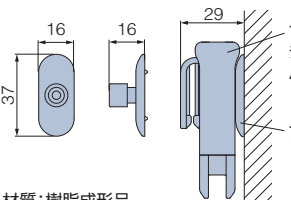
フック（壁付けの際に使用） [単位:mm]
