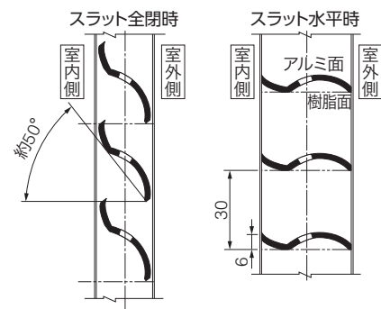
側面詳細図
