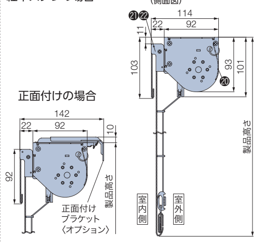
経木スダレの場合
