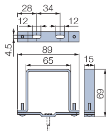
ワイヤープラケット※
