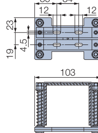
ワイヤーブラケット
