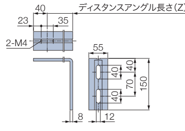
L型ブラケット(正面付けの場合に付属)
