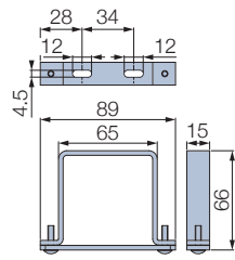
取付けブラケット
