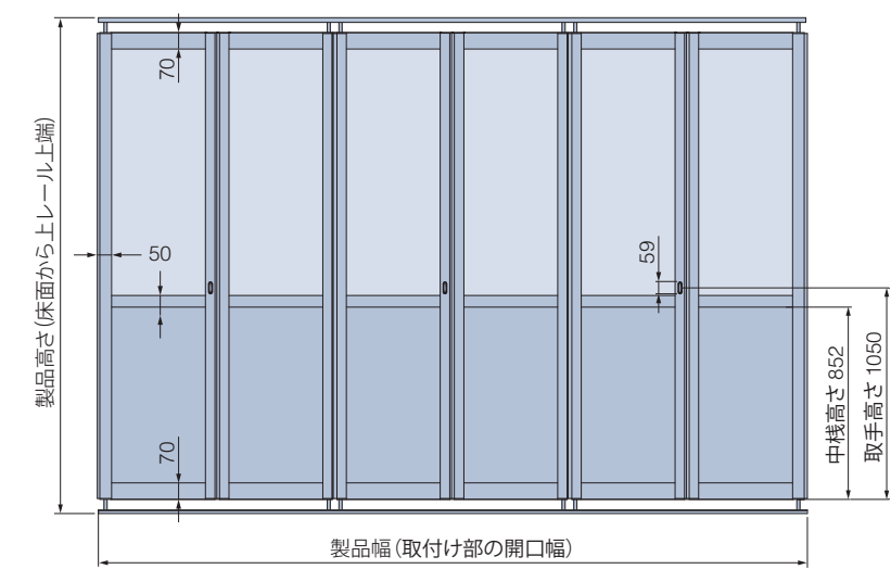
■ 正面図 *図は/パネルデザインB-2の場合
