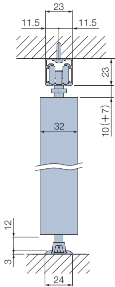
フラットガイドレール
