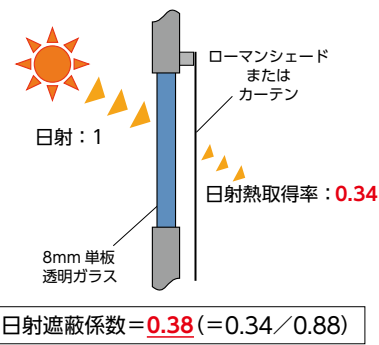
ガラス+ローマンシェードまたはカーテン(セーブス)の場合 [ガラス条件:8mm単板透明ガラス]
