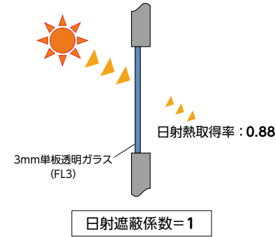
ガラスのみの場合 [3mm単板透明ガラス]
