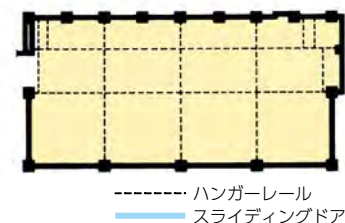
レール配置図
